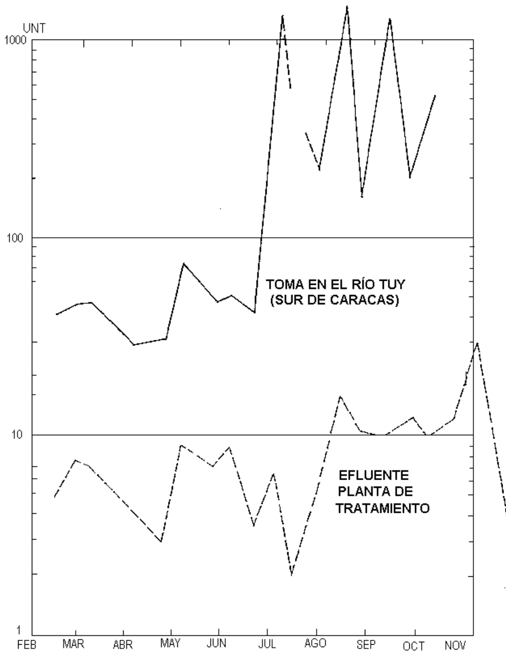
Figura 4.2 Variación de la turbiedad (muestra de 1996) UNT: Unidades nefelométricas de turbiedad
