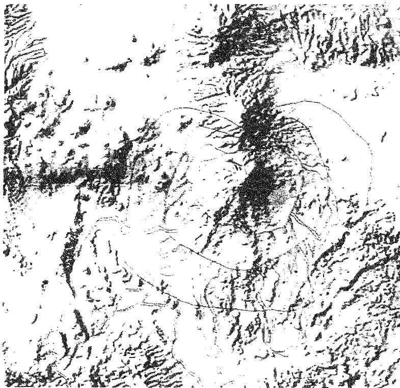
Fig. 5. Índice de aspecto de la pendiente.
