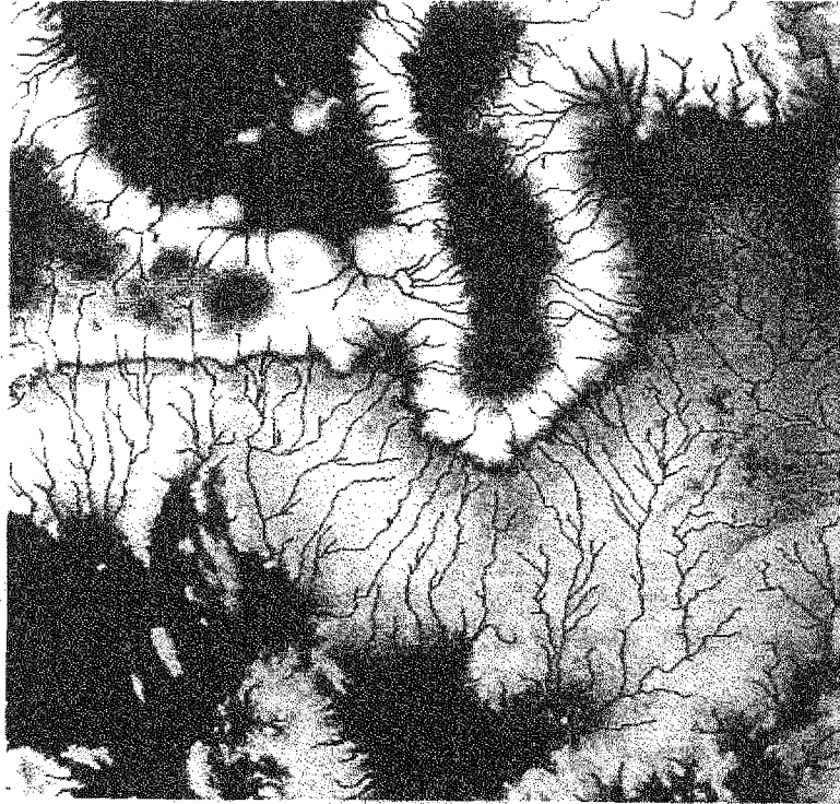
Fig. 4. Modelo de elevación del terreno con líneas de acumulación de flujo en negro.
