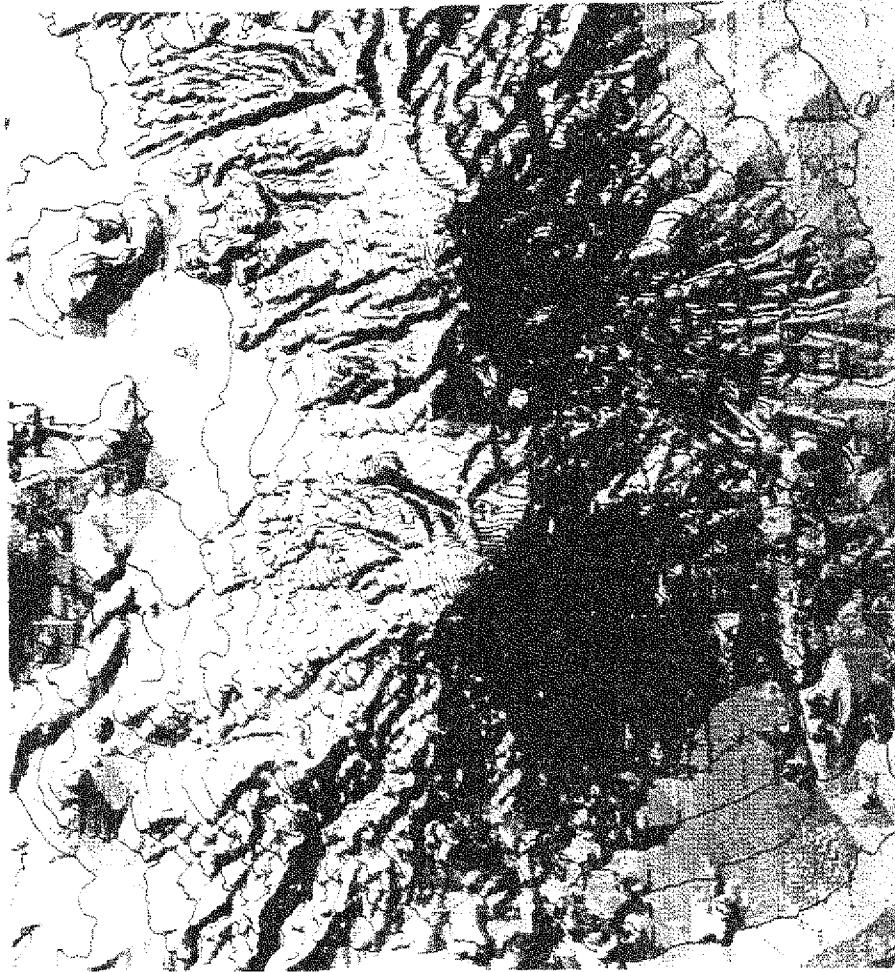
Fig. 6. Índice de aspecto de la pendiente con líneas de topografía superpuestas.
